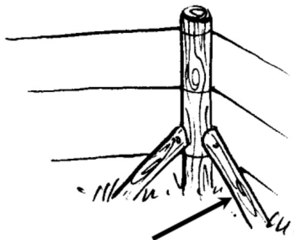
Die stut in die heining moet sterk en solied genoeg wees om die heining stabiel te maak.
