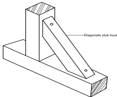
'n Diagonale stut in 'n hoek waar twee stukke hout bymekaarkom.
