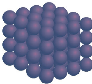
Die deeltjies in 'n vaste stof.
