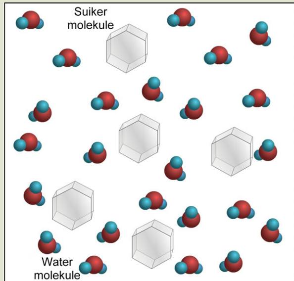
'n Oplossing van water- en suikermolekule (deeltjies)
