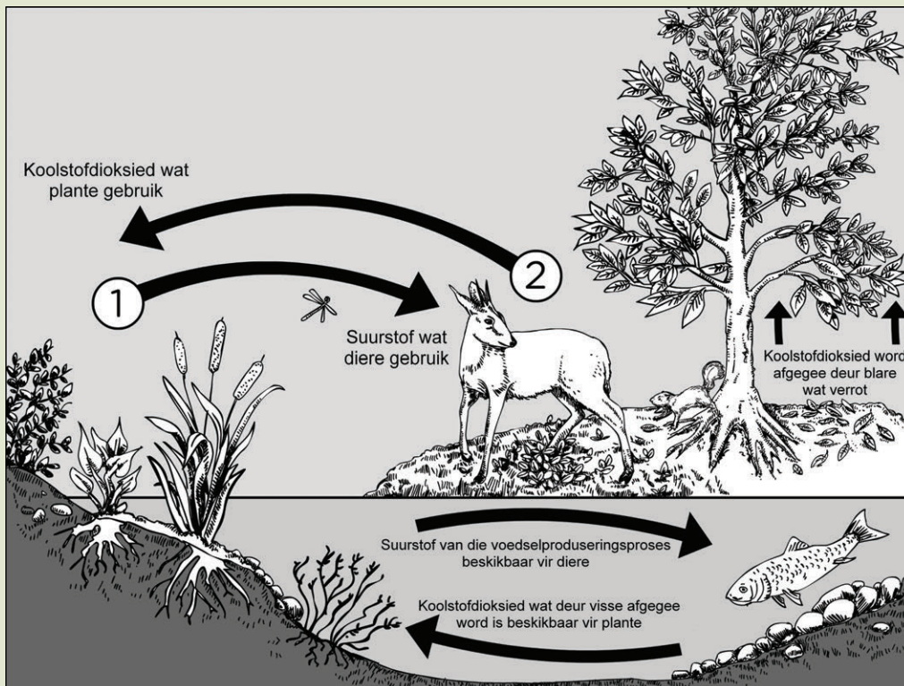
Die suurstof- en koolstofdioksiedsiklus.
