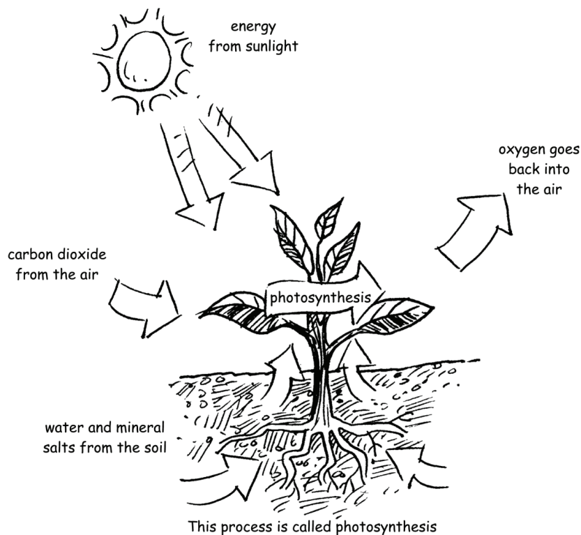
Die proses van fotosintese.
