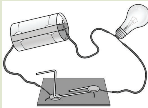
Die opstel van 'n skakelaar en 'n eenvoudige stroombaan.
