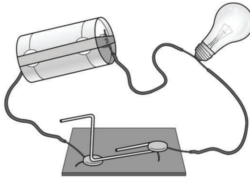
'n Skets van die eenvoudige stroombaan met 'n skuifspeldskakelaar, battery en gloeilamp.
