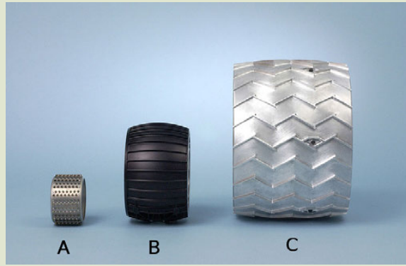
Die wiele van drie Marsmaantuie.
