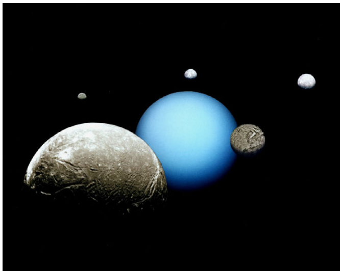
Die blou bol Uranus, met 5 van sy grootste mane.
