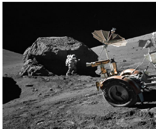
Ruimtevaarder Schmitt versamel monsters op die maan.
