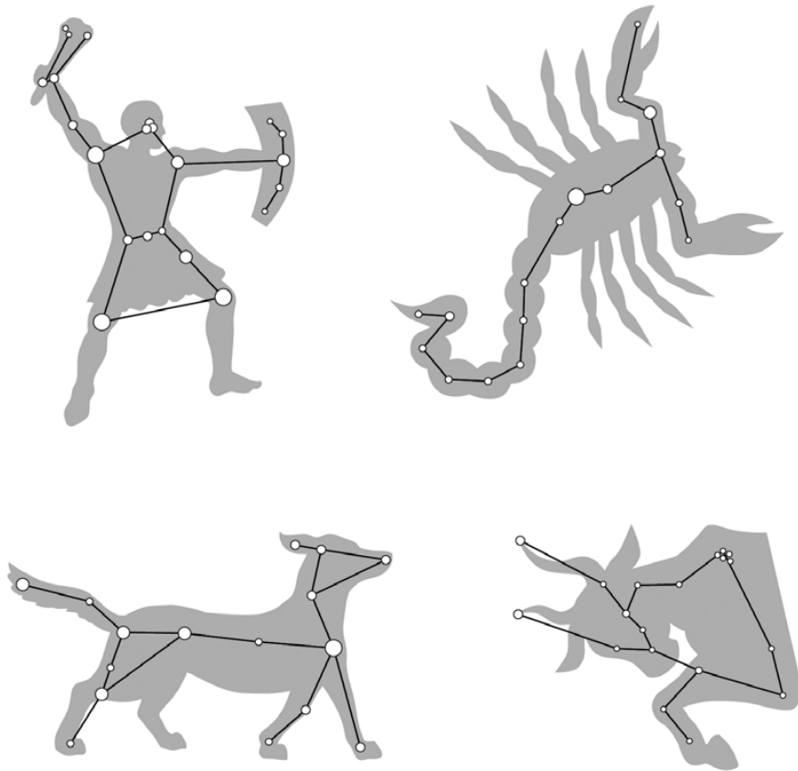
Sommige konstellasies van sterre maak patrone in die lug.
