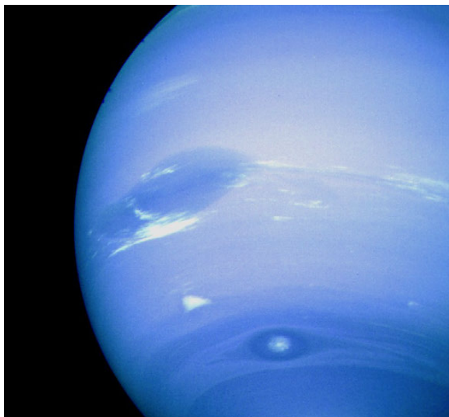
'n Naby-beeld van die oppervlak van Neptunus. Kan jy die stormagtige oppervlakte sien? Dit is die donkerblou en wit kolle.
